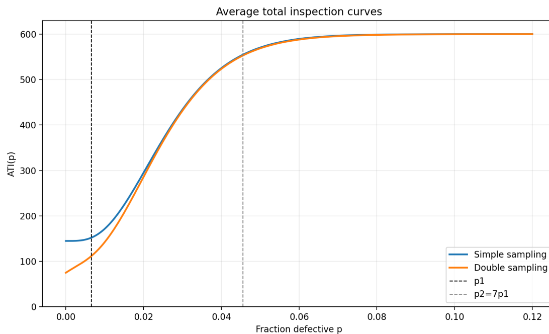
Σχήμα 2: Μέσος συνολικός αριθμός επιθεωρούμενων μονάδων ATI(p) .
