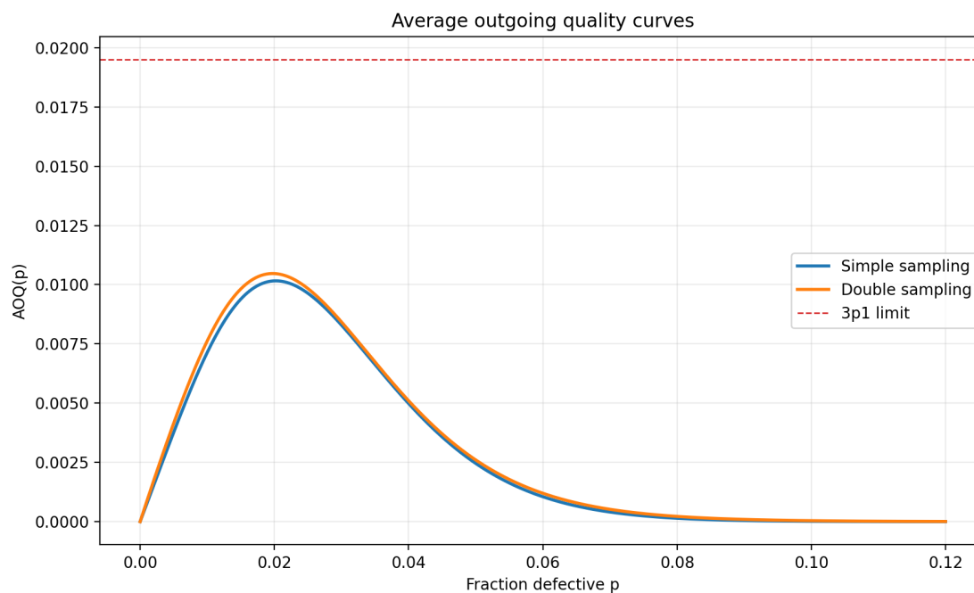
Σχήμα 3: Μέση εξερχόμενη ποιότητα AOQ(p) και όριο 3p_1 .
